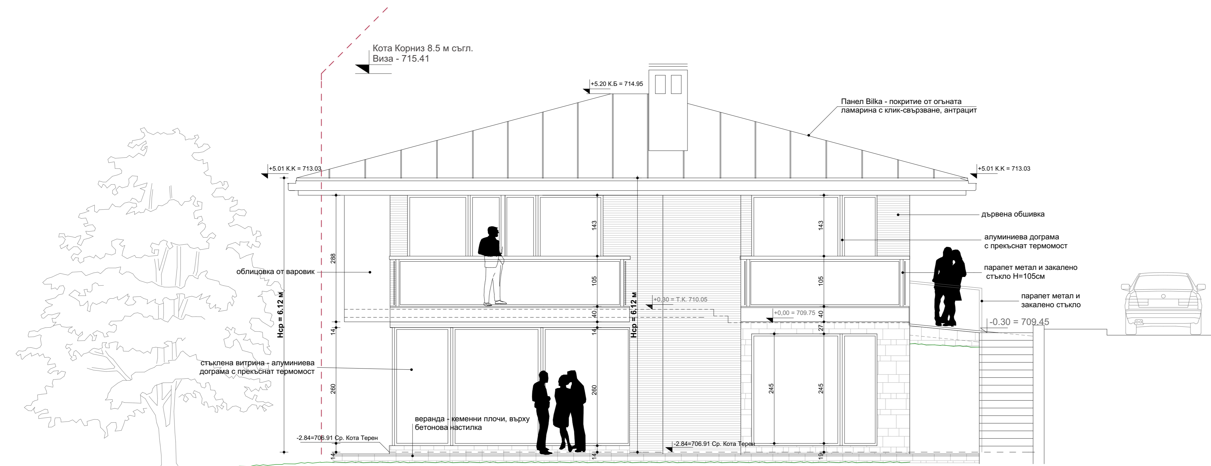
ФАСАДА ЗАПАД МАЩАБ 1:50
