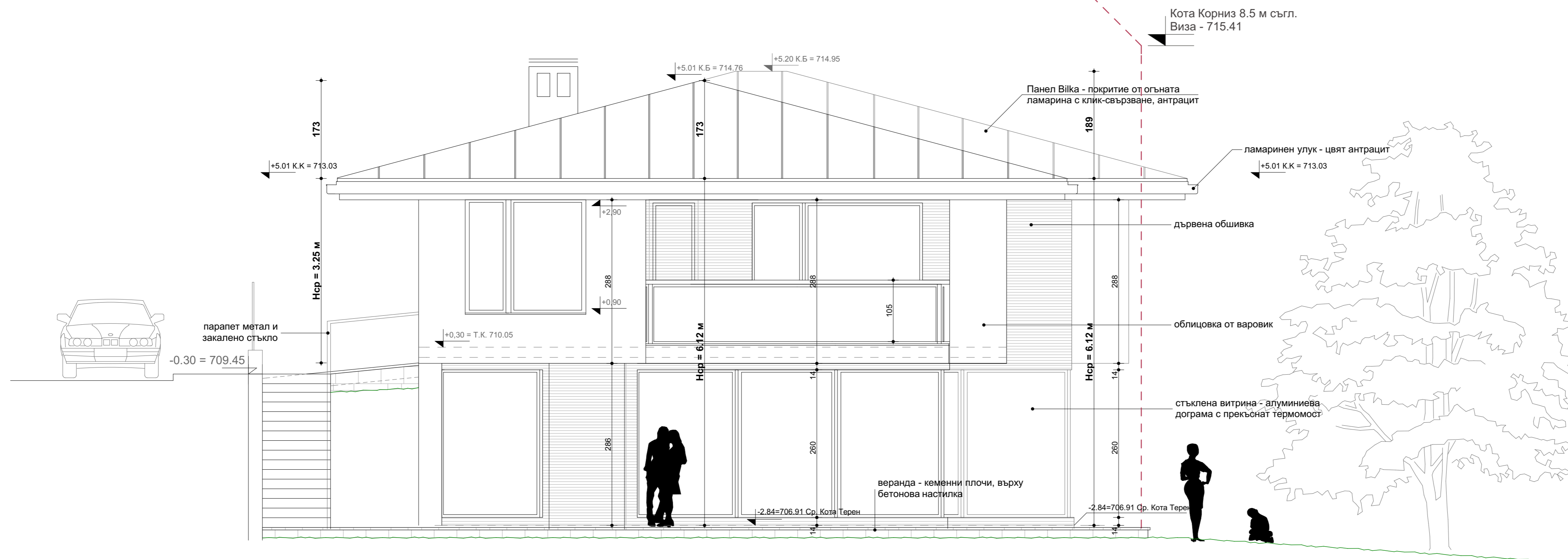
ФАСАДА ИЗТОК МАЩАБ 1:50
