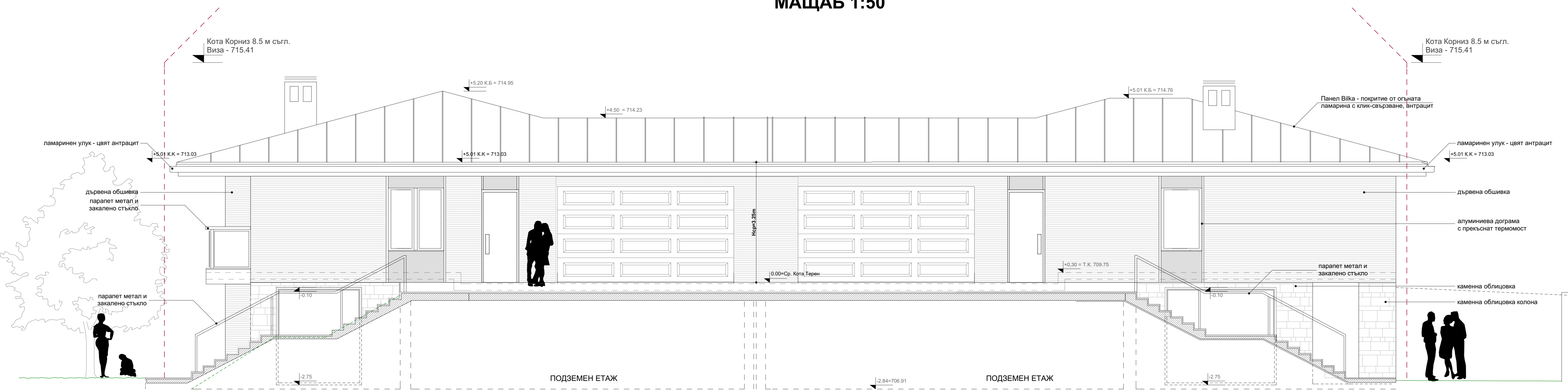
ФАСАДА ЮГ МАЩАБ 1:50
