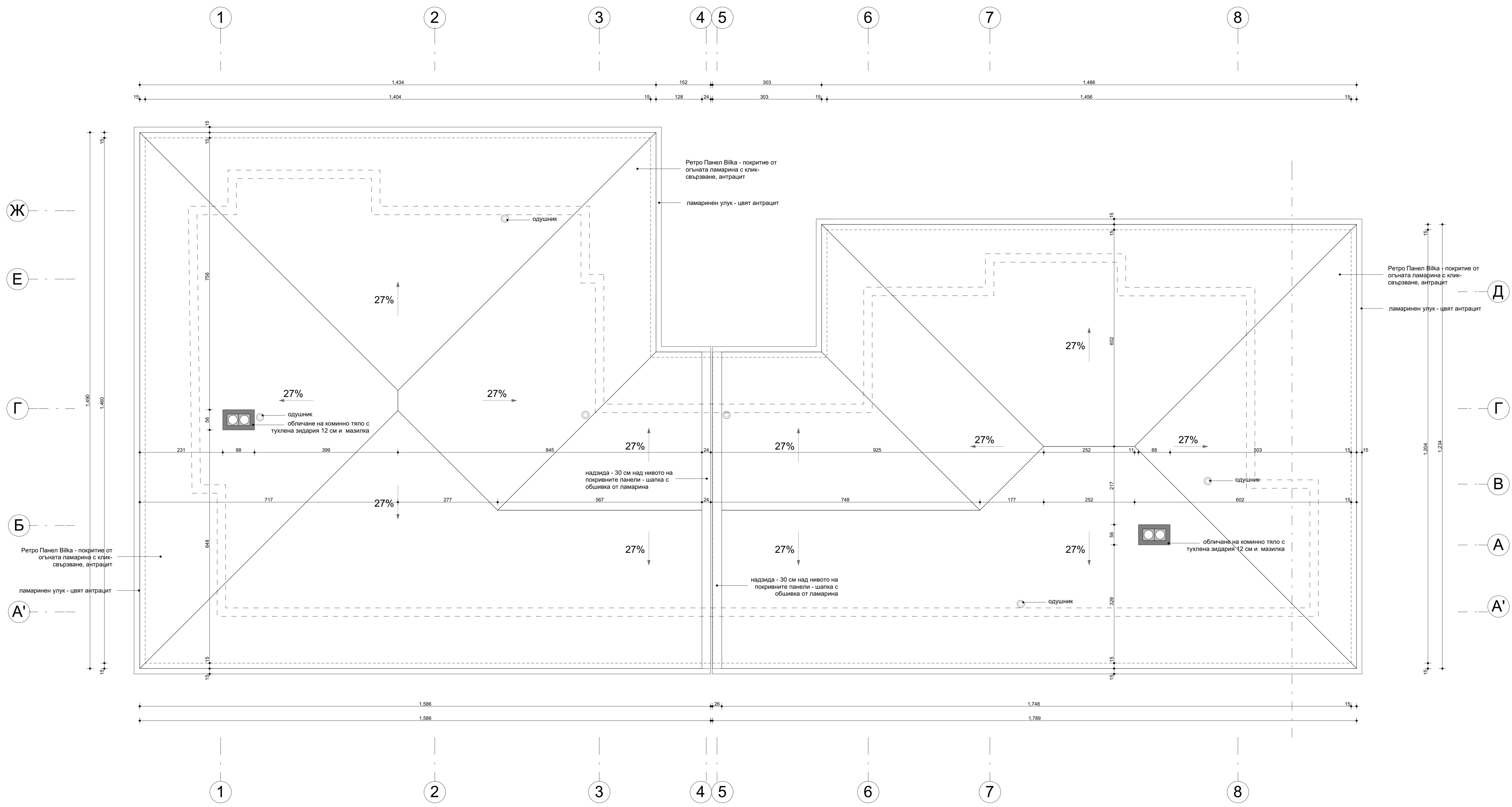
ПЛАН ПОКРИВ МАЩАБ 1:50
