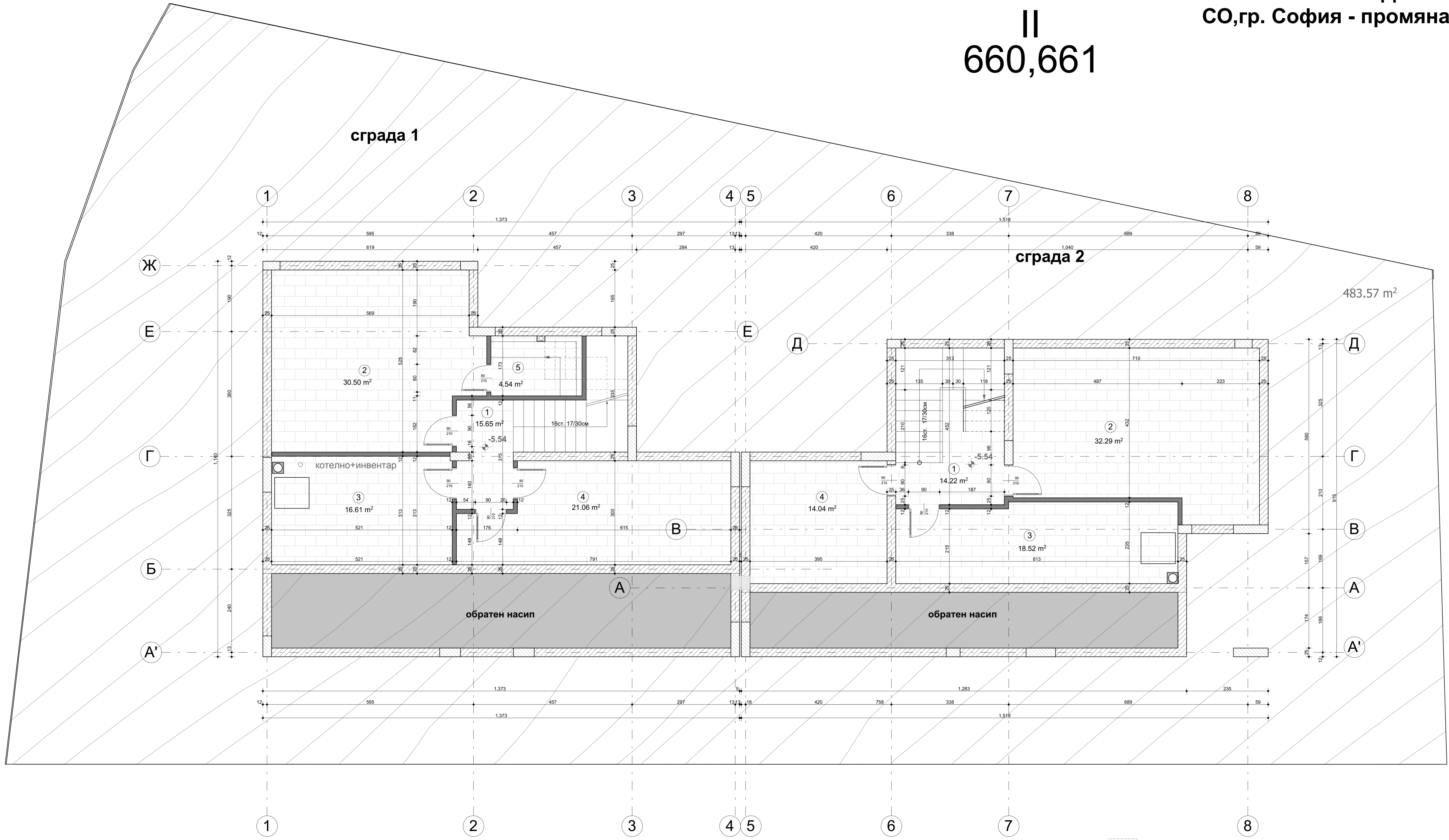
РАЗПРЕДЕЛЕНИЕ СУТЕРЕН / КОТА -5.87 МАЩАБ 1:50
